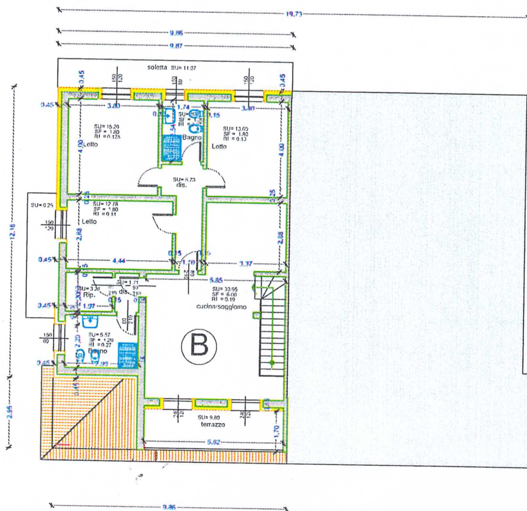
pianta piano primo unità B
